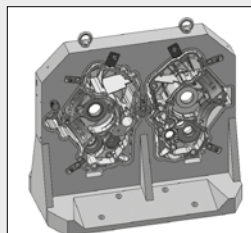
Mechanický upínací přípravek
